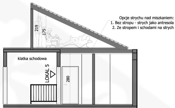
PRZEKRÓJ MIESZKANIA NR 5
