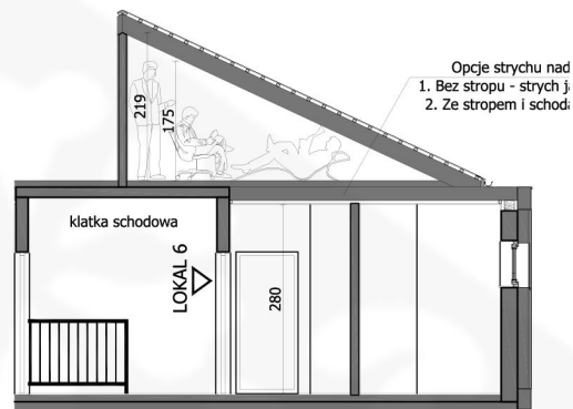
PRZEKRÓJ MIESZKANIA NR 6
